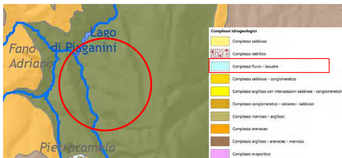
Complessi idrogeologici nell'ambito di Fano Adriano
